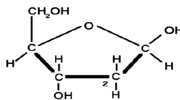
2-désoxy- \beta -D-Ribose
