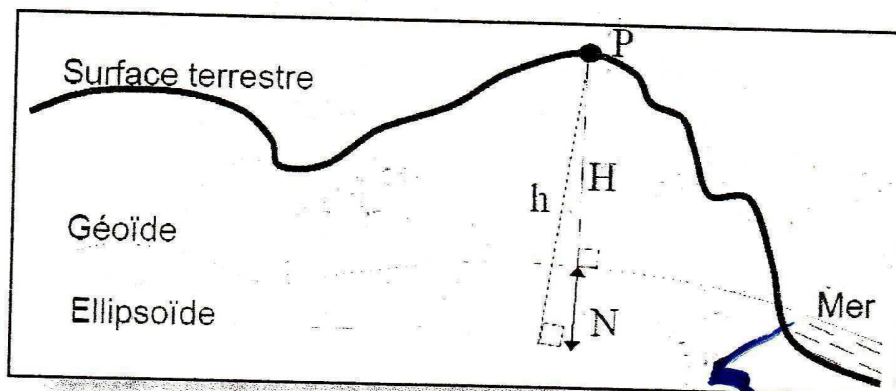
Figure 3 : Définition de la position d'un point sur la surface topographique selon le géoïde et l'ellipsoïde (CAVAYAS .F, 2011).
