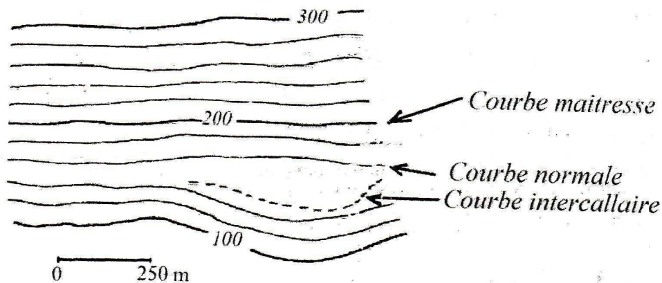
Figure 6 : Différents types de courbes de niveau
