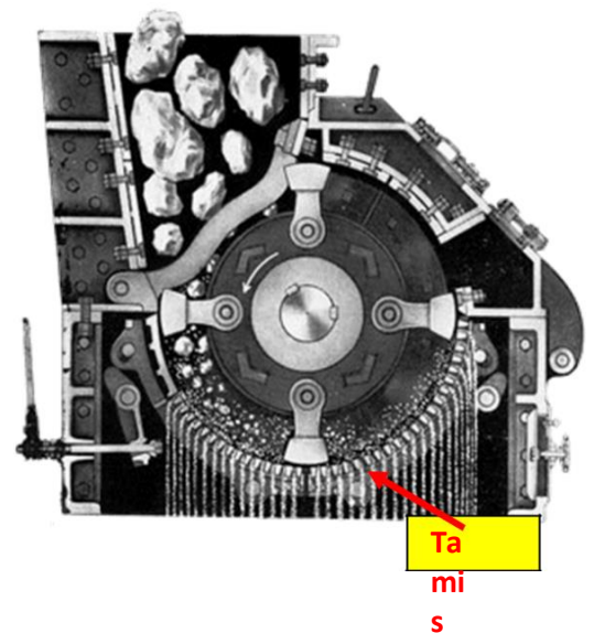
Concasseur à marteaux
