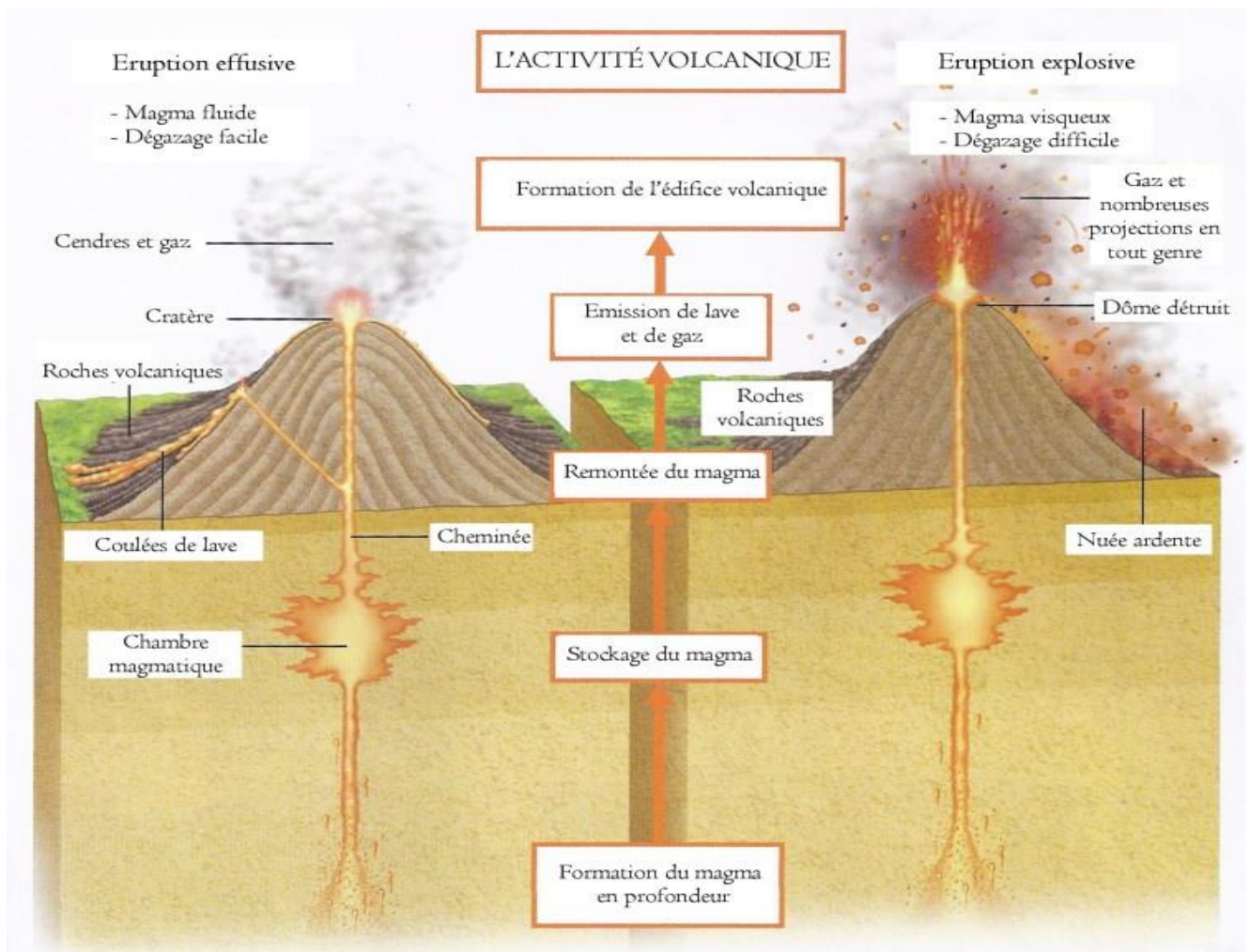
Figure.10. Types d'éruptions volcaniques
