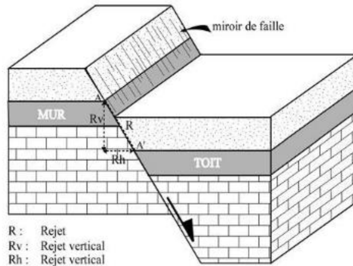
Figure.04. Structure faillée
