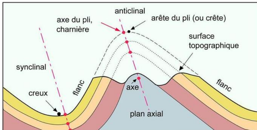
Figure.06. structure plissée
