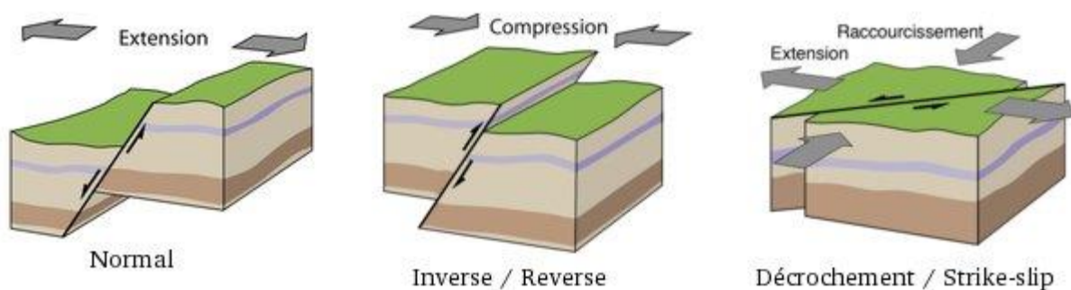
Figure.05. Différents types de failles
