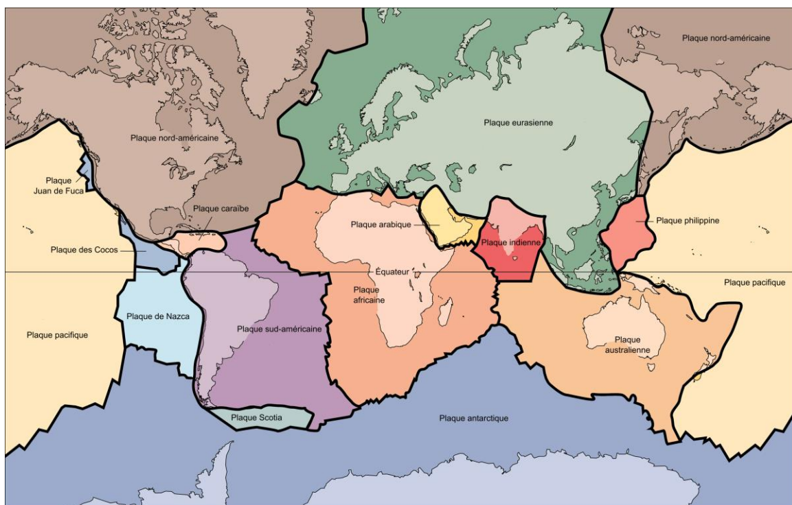
Figure.12. carte des principales plaques tectoniques terrestres.
