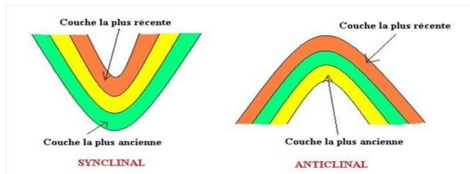
Figure.07. anticlinaux et synclinaux
