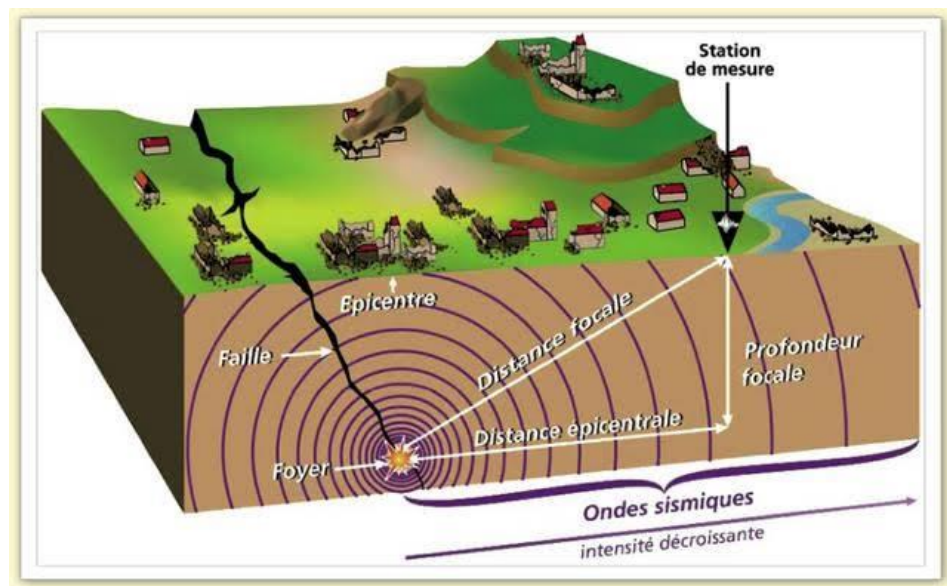
Figure.01. Caractéristiques générales d'un séisme
