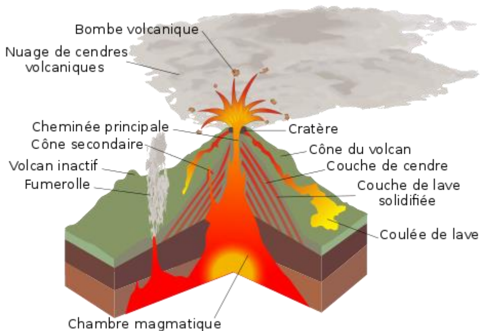
Figure.09. Structure typique d'un volcan
