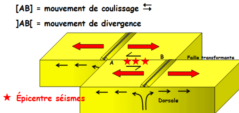
Figure.15. les failles transformantes.
