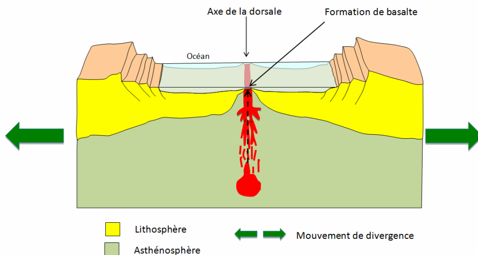
Figure.13. zones d'accrétion océanique (dorsales océaniques)
