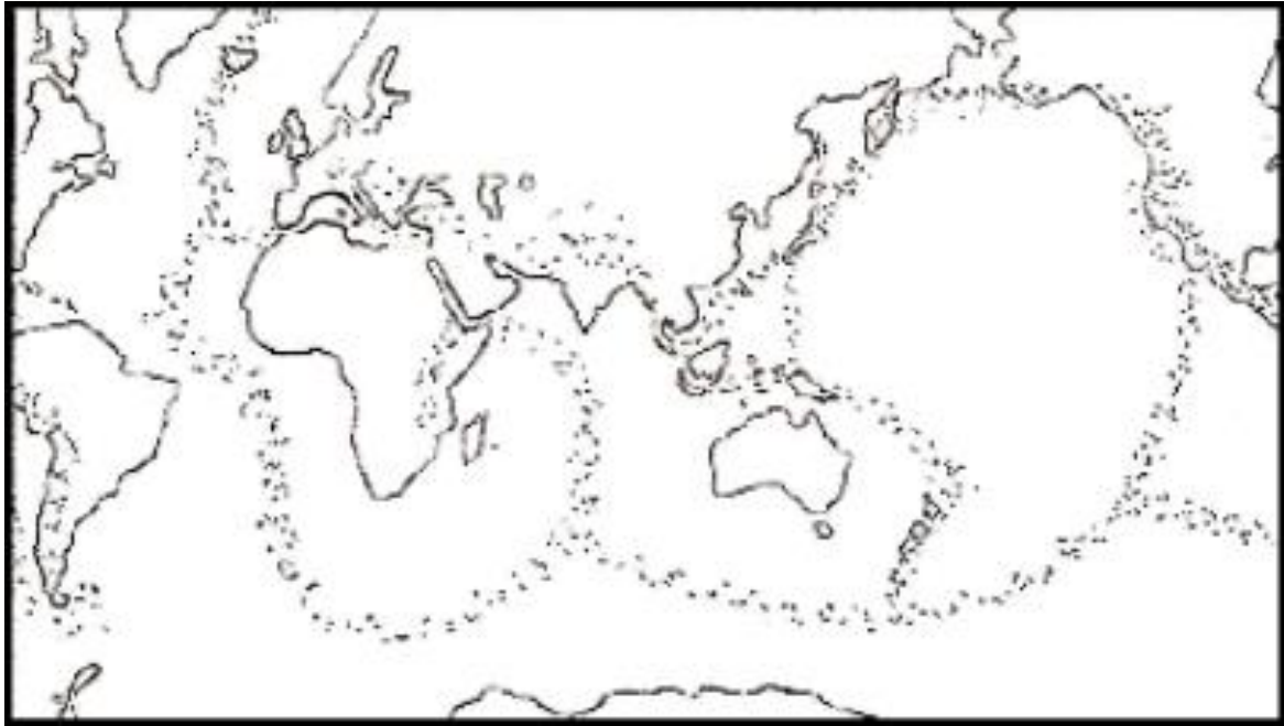
Figure.02. localisation des séismes dans le monde
