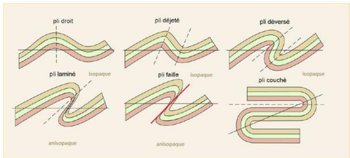
Figure.08. les plis isopaques et les plis anisopaques
