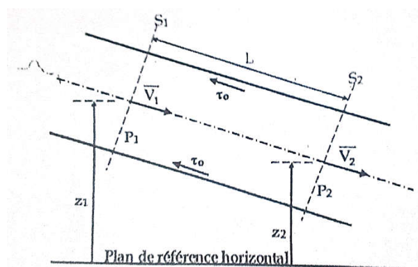
Fig. 4 : Caractéristiques d'un écoulement dans un tronçon de conduite rectiligne et de section droite circulaire et constante.
