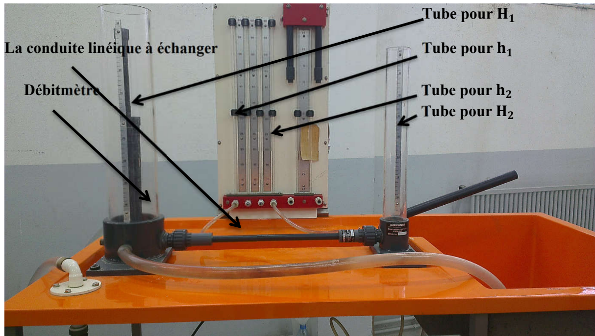
Fig. 8 : Banc d'essais
