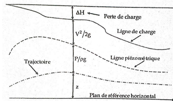
Fig. 5 : Représentation graphique de l'équation de Bernoulli dans le cas d'un liquide réel
