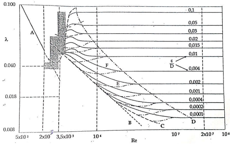
Fig. 6 : Diagramme de Moody.
