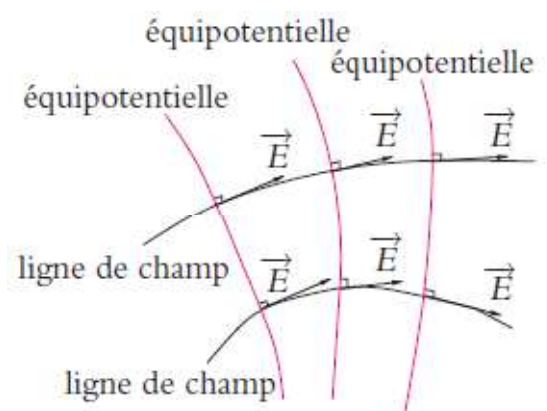
Figure 16.5 Lignes de champ normales aux équipotentiels
