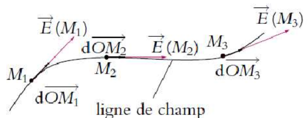
Figure 44.11 Définition d'une ligne de champ.
