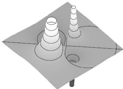
Figure 44.15 Équipotentiellles d'une distribution discrète de quatre charges. Le niveau de gris traduit l'intensité relative du potentiel.
